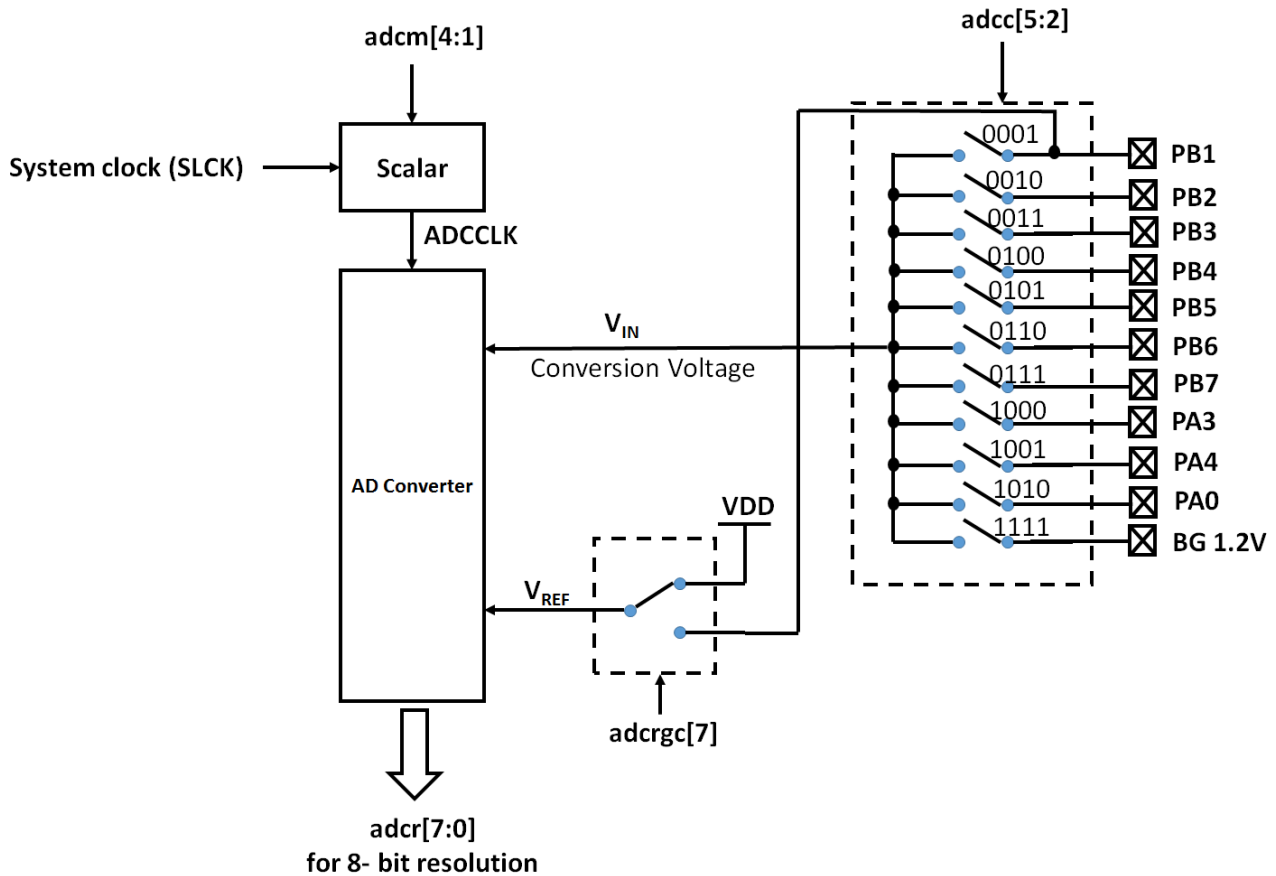
图 19: ADC 模块框图
