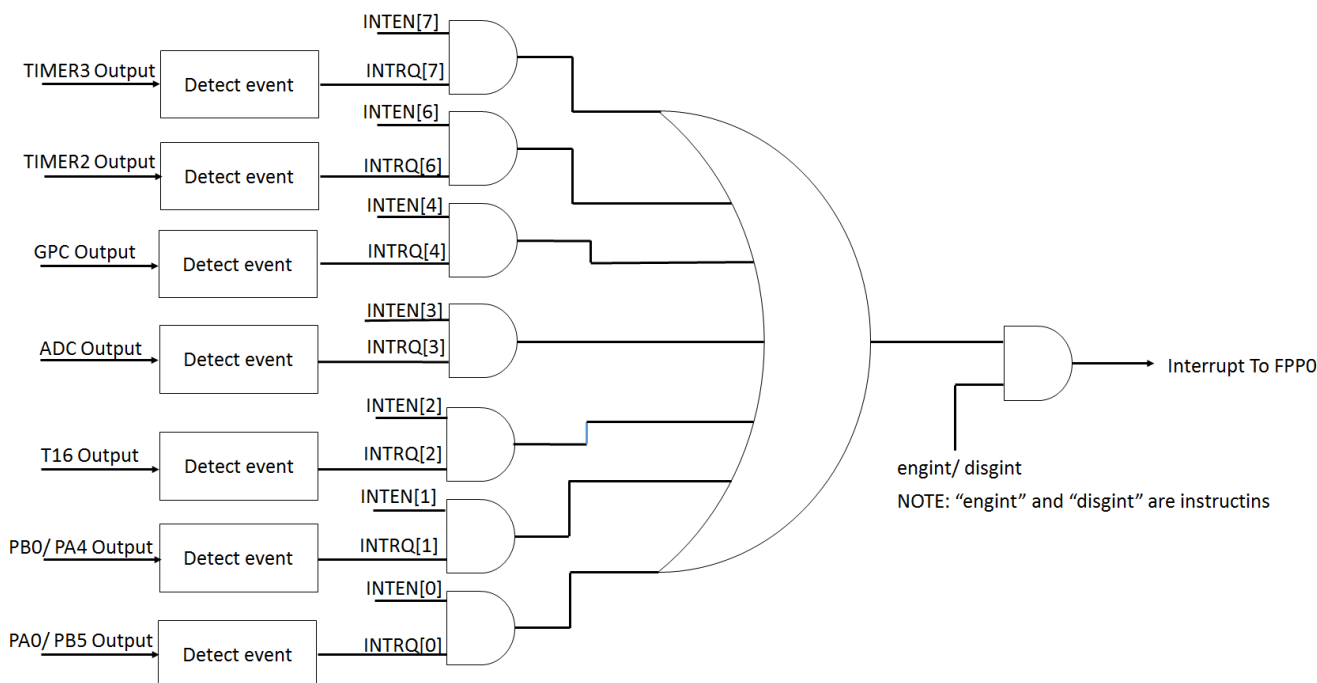
图 16: 中断控制器硬件框图
