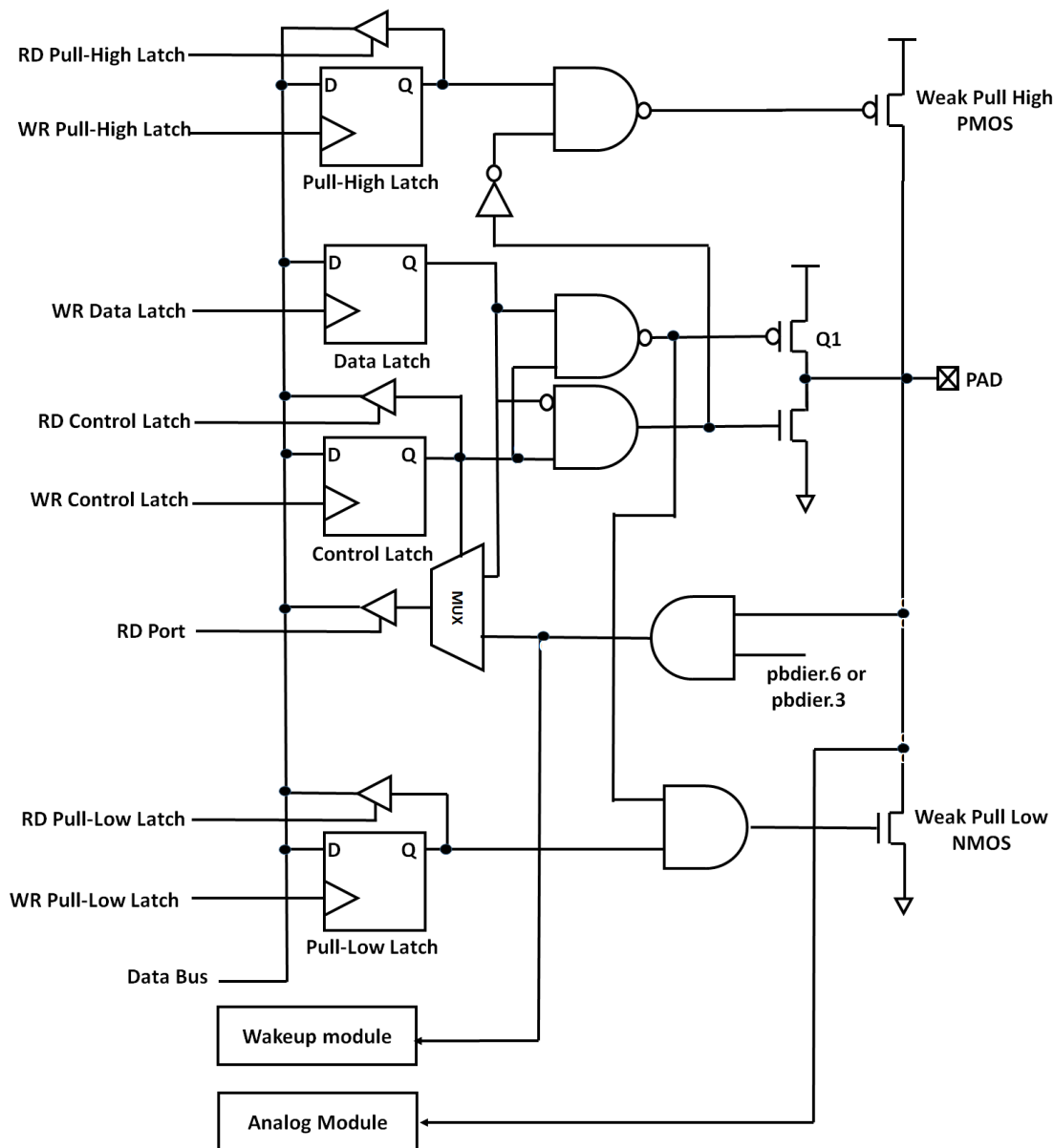
图 18: 带弱上拉电阻和弱下拉电阻的 IO 引脚缓冲区硬件图
