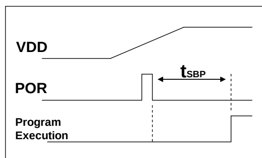
图 1：上电复位时序
