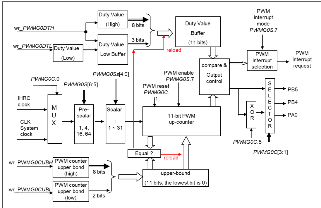
图 15: 11 位 PWM 生成器硬件框图
